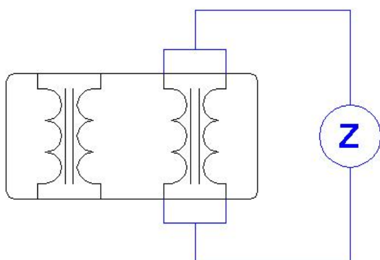
(A):Common mode
